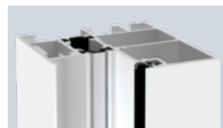
Sarkos kivitel (A2 profil)
